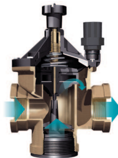
BPES Schnittdarstellung
