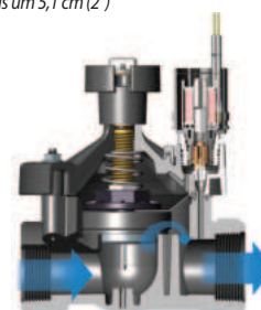
PEB Schnittdarstellung
