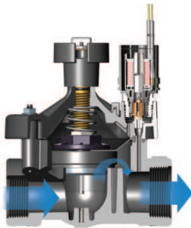
PEB Schnittdarstellung
