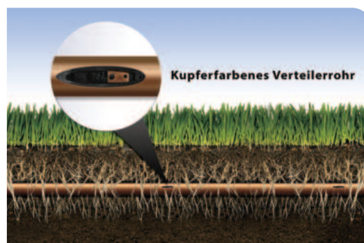
Unterirdisches XFS-Tropfrohr mit Copper Shield™-Technologie
