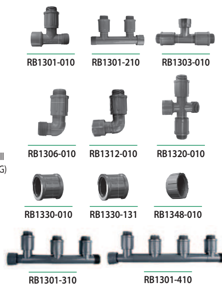
TYPENREIHE RB 1300
