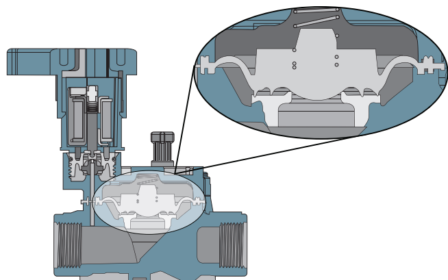
Einzigartiges Membrandesign
