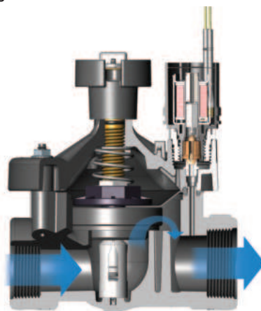
PESB Schnittdarstellung
